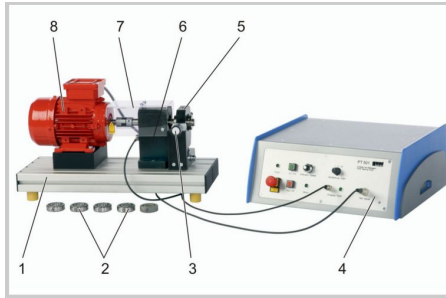
1 plaque de fondation, 2 palier à roulement, 3 dispositif de charge, 4 appareil de commande, 5 accueilli du palier à étudier, 6 logement de l'arbre, 7 couvercle transparent, 8 moteur.
