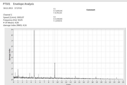
Analyse d'enveloppe d'un palier à roulement avec dommages sur le joint torique externe (B) à 6-3000min -1
