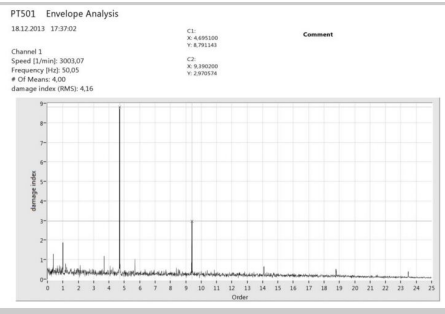
Analyse d'enveloppe d'un palier à roulement avec dommages sur le joint torique externe (B) à n=3000\text{min}^{-1}
